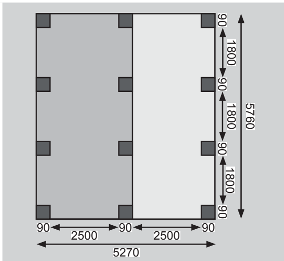
Carport + Abstellraum 3
